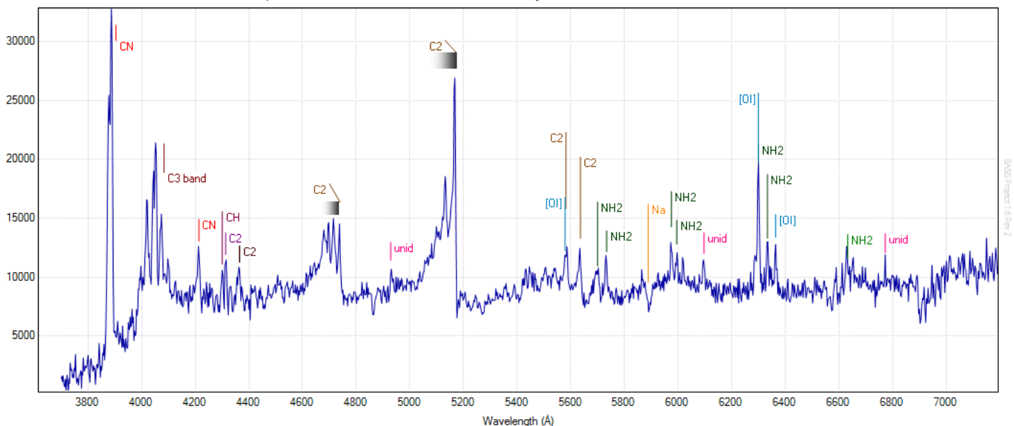
COMETA LOVEJOY - DADOS 200l/mm ; C11 ; Atik 314L + ; Tejina (Tenerife)
