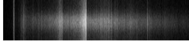
Espectro 200 l/mm C 2014 Q2
