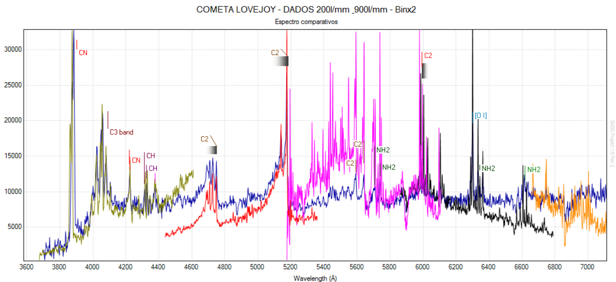
Conjunto comparativo de espectros obtenidos del Cometa Lovejoy a 900 l/mm sobre el mismo a 200 l/mm en azul.
