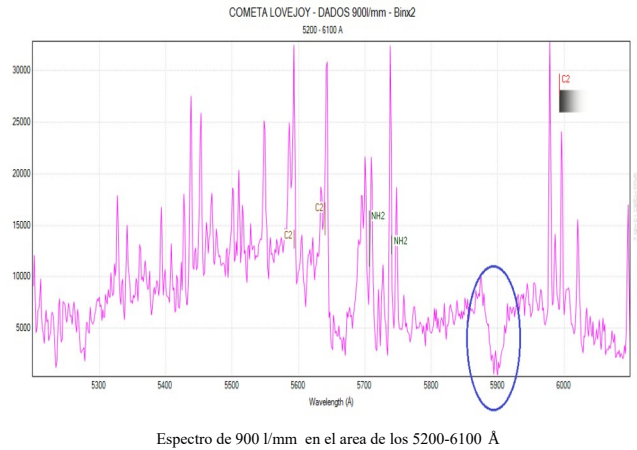
Espectro de 900 l/mm en el area de los 5200-6100 Å
