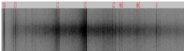
Espectro de 200 l/mm C 2014 Q2. AESAS,2015
